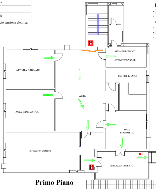
Figura 2. Pianta Emergenza Piano Primo Scuola Infanzia "Chiugiana"
