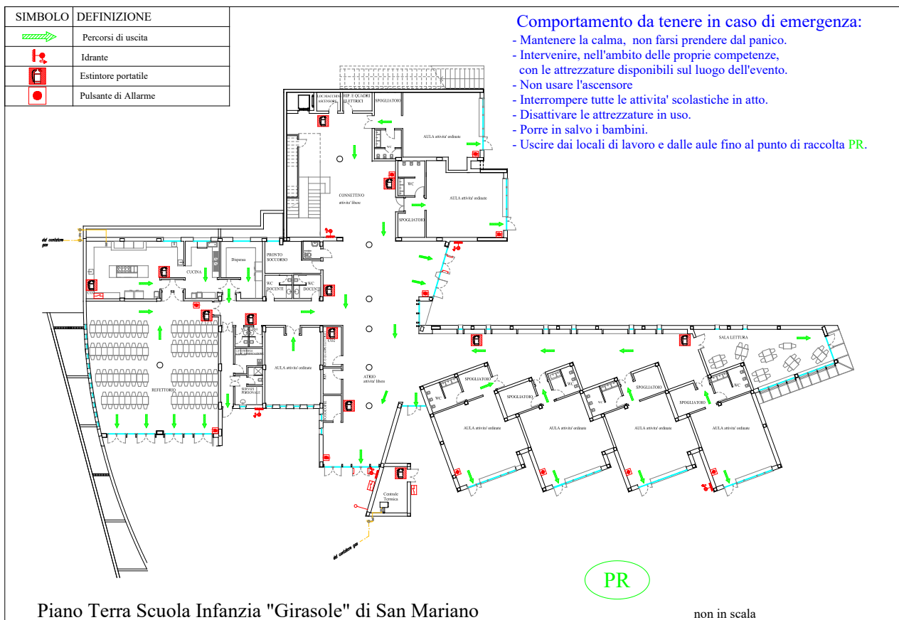
Figura 1. Pianta Emergenza Piano Terra Scuola Infanzia "Girasole"
