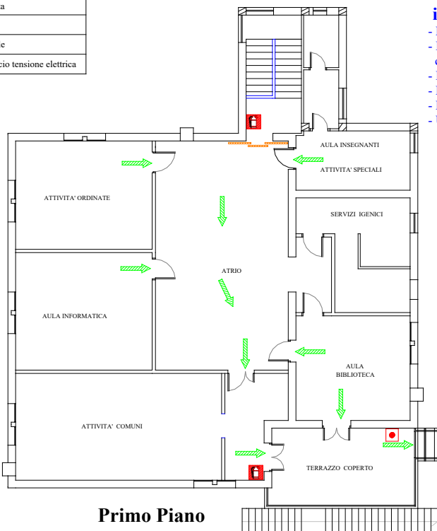
Figura 2. Pianta Emergenza Piano Primo Scuola Infanzia "Lucina" – San Mariano
