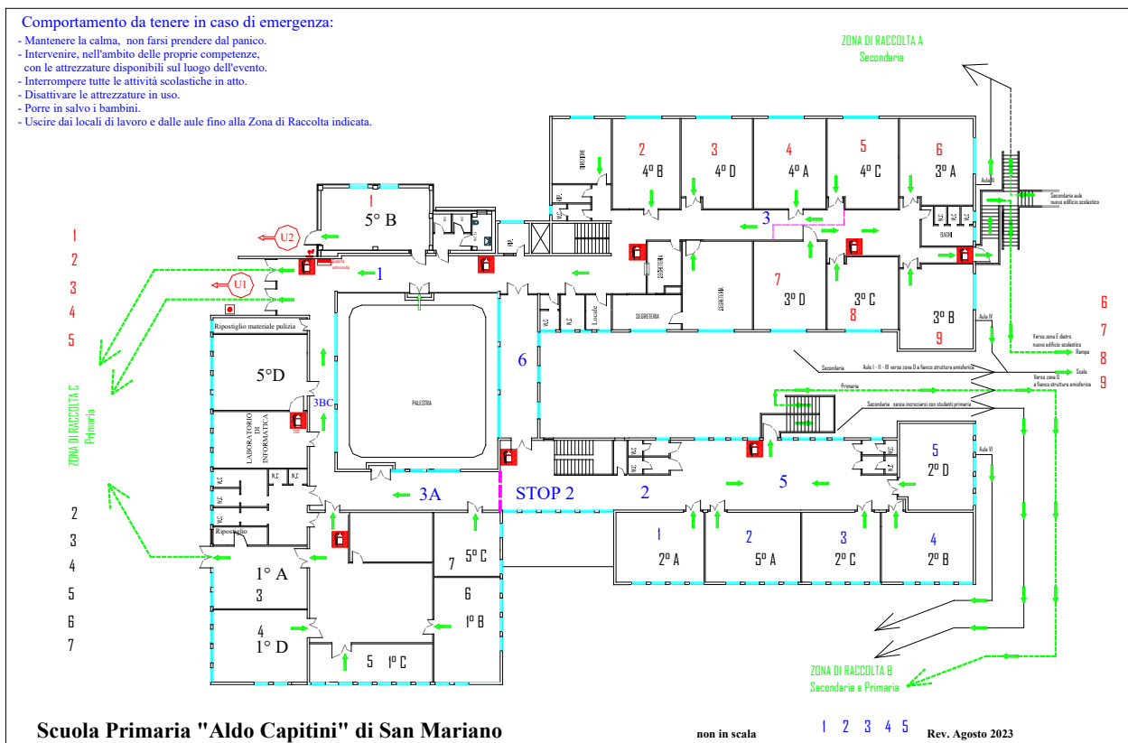
Figura 1. Pianta Emergenza Piano Scuola Primaria San Mariano
