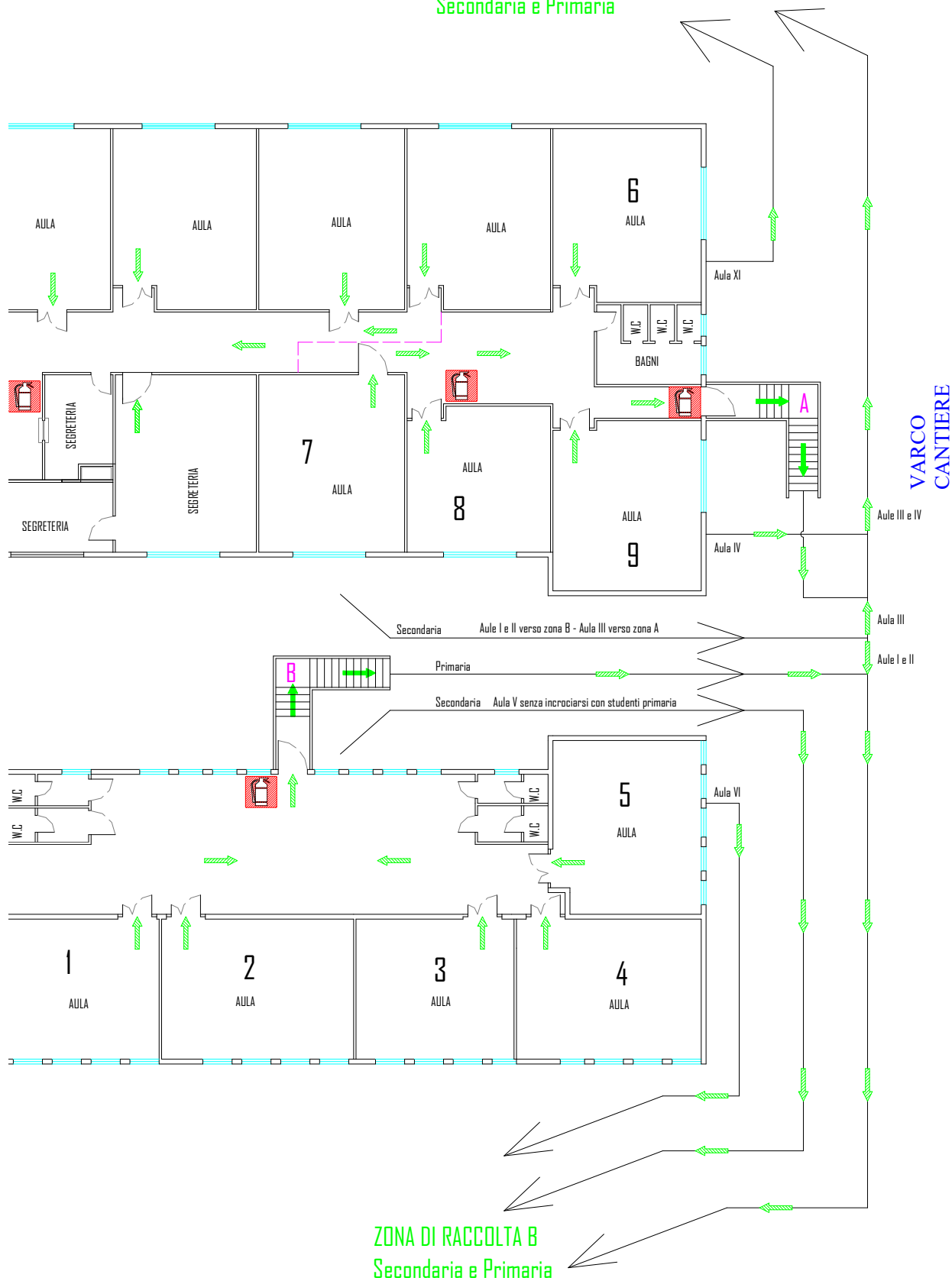
Figura 2. Procedura di Emergenza (percorso di evacuazione) Scuola Primaria San Mariano
